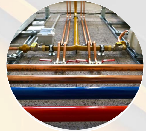
Instalación redes
